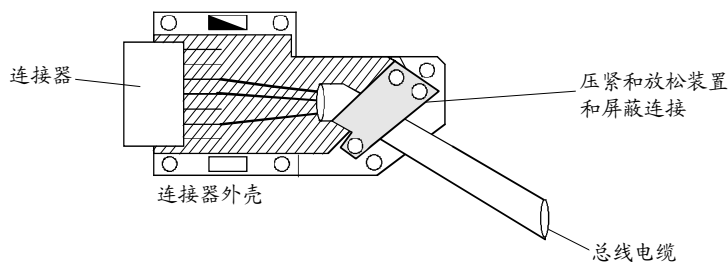
图 8.4-8 连接总线电缆
