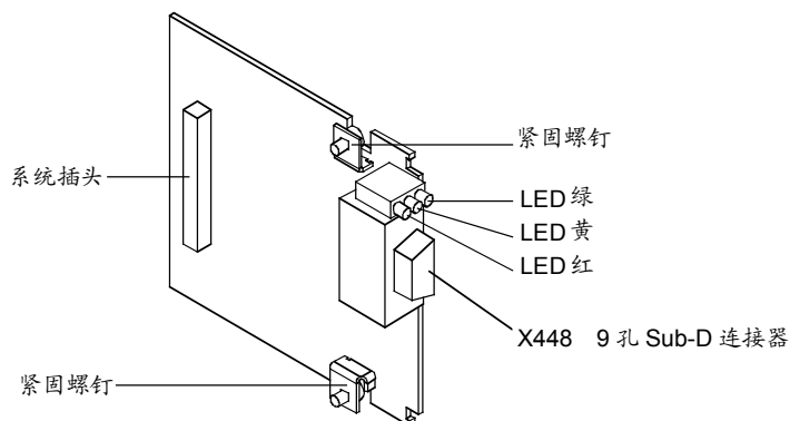
图 8.2-1 通讯板
