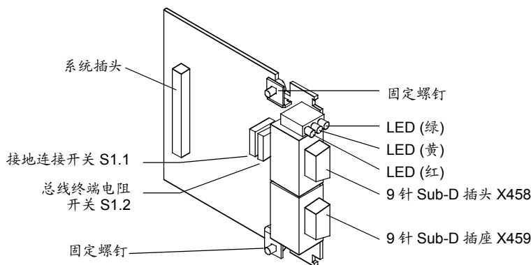
图 8.4-1 选件 CBC 板视图
