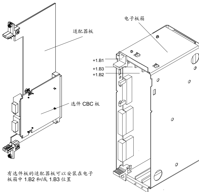
图 8.4-6 具有空插槽(+1.B2 和+1.B3)和带 CBC 的适配器板的电子箱
