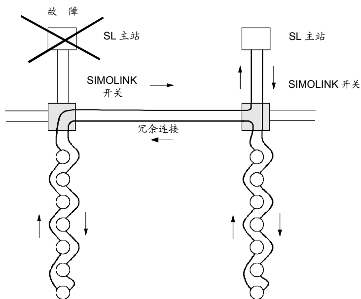
图 8.3-1 SIMOLINK 开关应用示例
