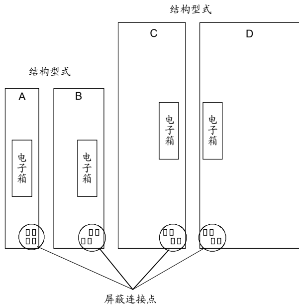
图 8.4-10 屏蔽连接点的位置
