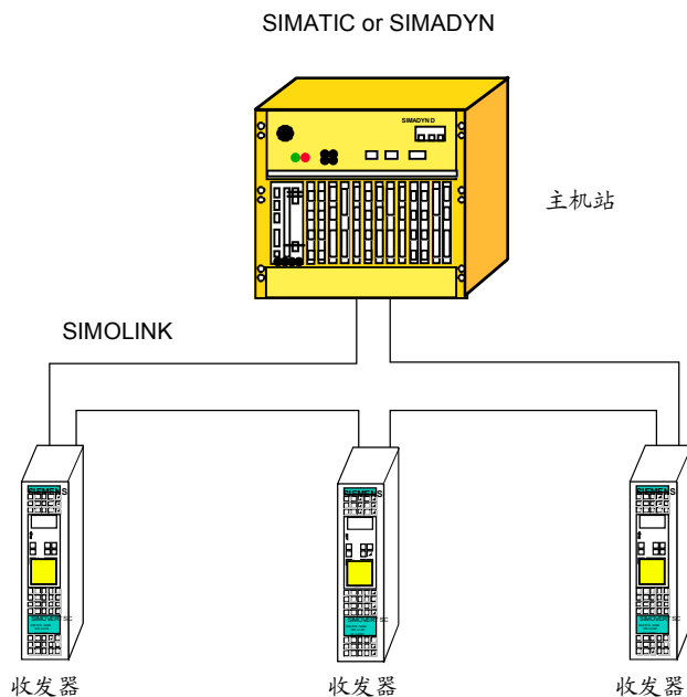
图 8.3-13 主/从功能应用示例
