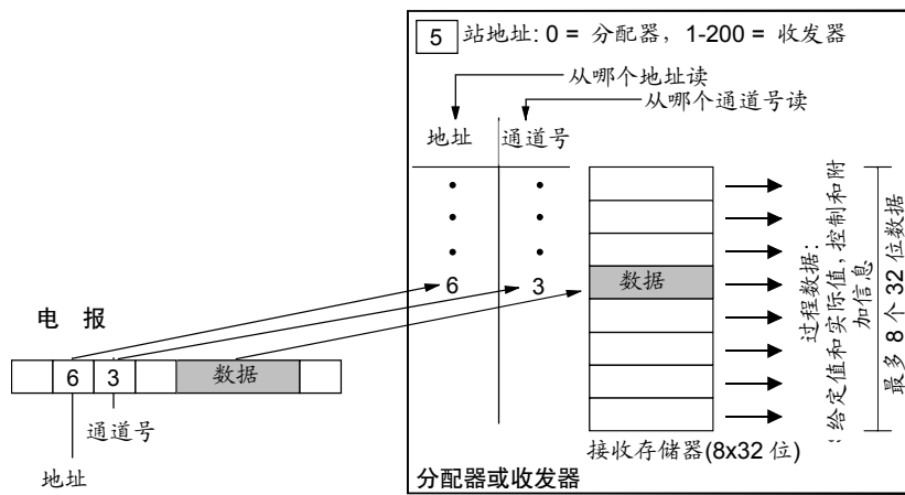
图 8.3-5 读数据
