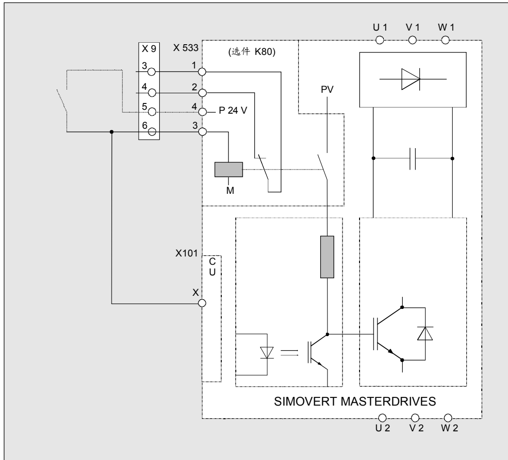
图 2-10 在一台 SIMOVERT MASTERDRIVES 装置中 “安全停车”功能的配置
