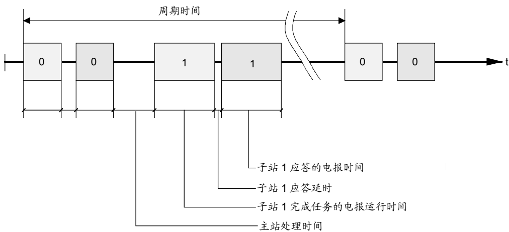
图 8.1-5 周期时间
