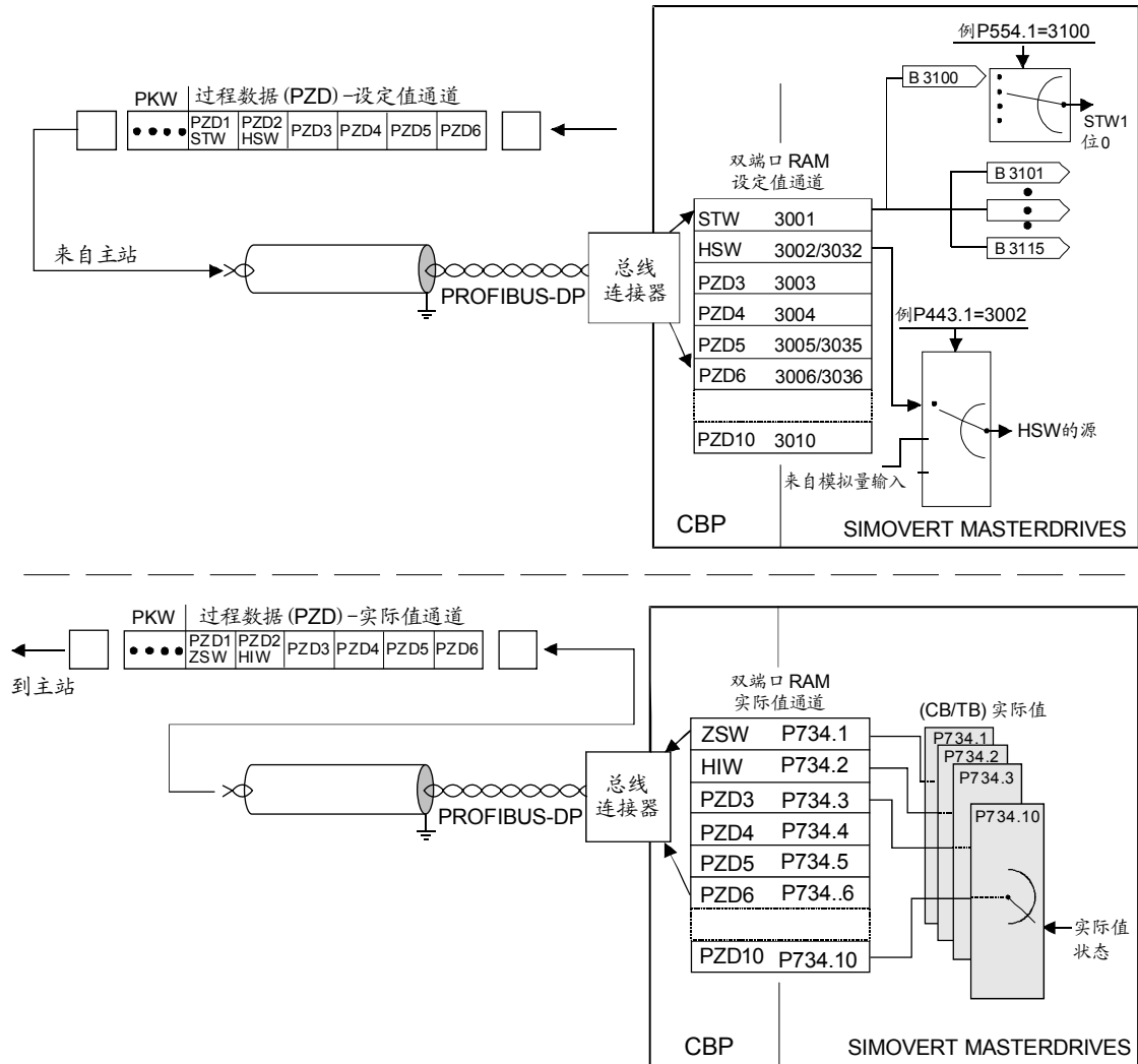
图 8.2-21 第一个 CB 板用于功能类 Motion control Compact PLUS, CUPM, CUMC 和 CUVc 过程数据互连的例子
