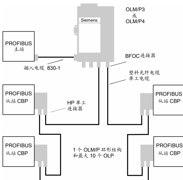
图 8.2-15 用 OLPs 系统配置的例子
