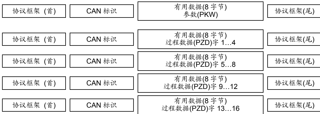
图 8.4-2 CAN 协议电报中的有用数据结构
