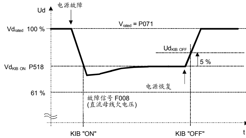
图 7-2 开关阈值
