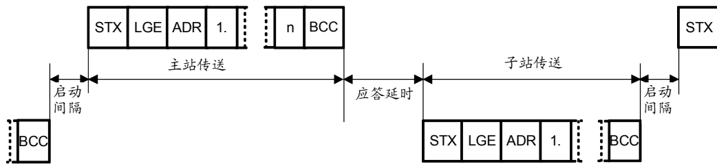
图 8.1-6 传送顺序
