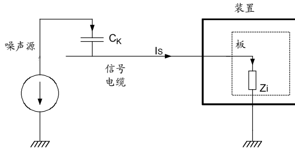
图 3-5 无屏蔽信号电缆的容性耦合
