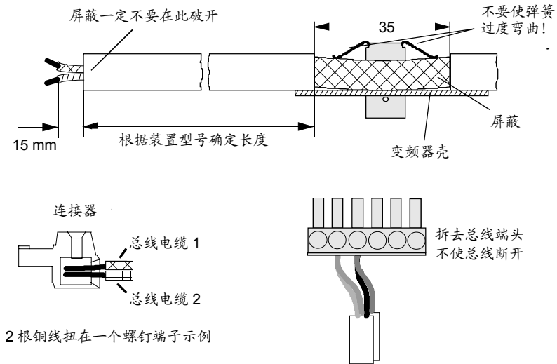
图 8.1-9 总线电缆的连接
