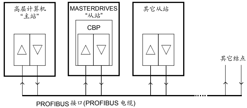
图 8.2-2 PROFIBUS 接口
