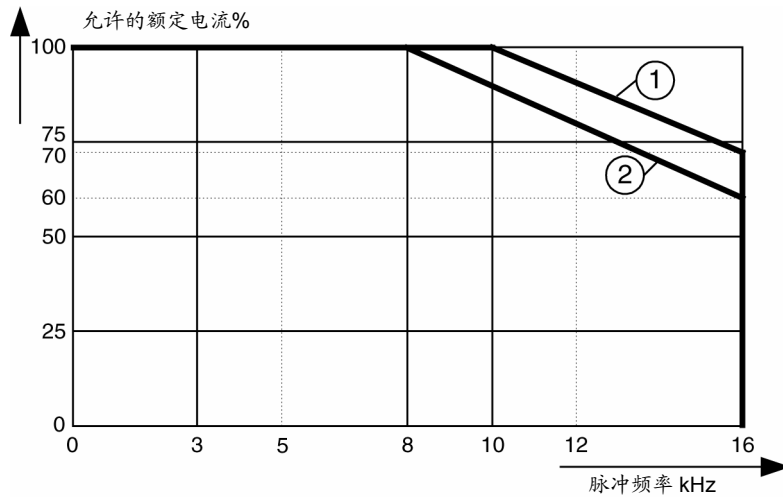
图 7-7 降额曲线
