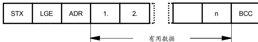
图 8.1-2 电报结构
