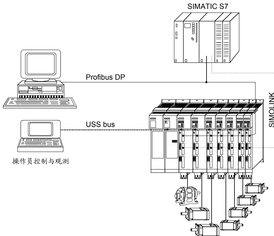
图 8-1 通讯一览
