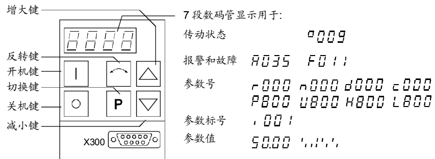
图 5-4 PMU 参数设置单元
