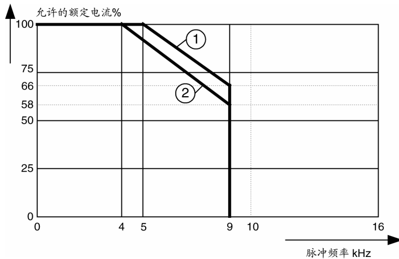
图 7-8 降额曲线
