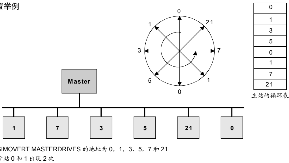
图 8.1-4 循环表
