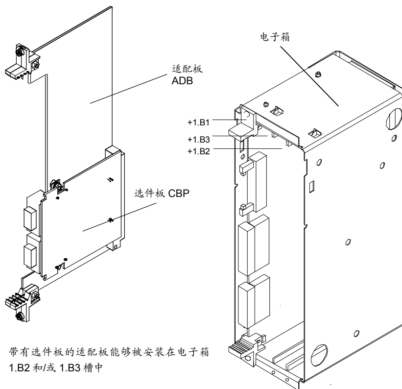
图 8.2-10 带有空槽(+1.B2 和 +1.B3)的电子箱和带有CBP的适配器
