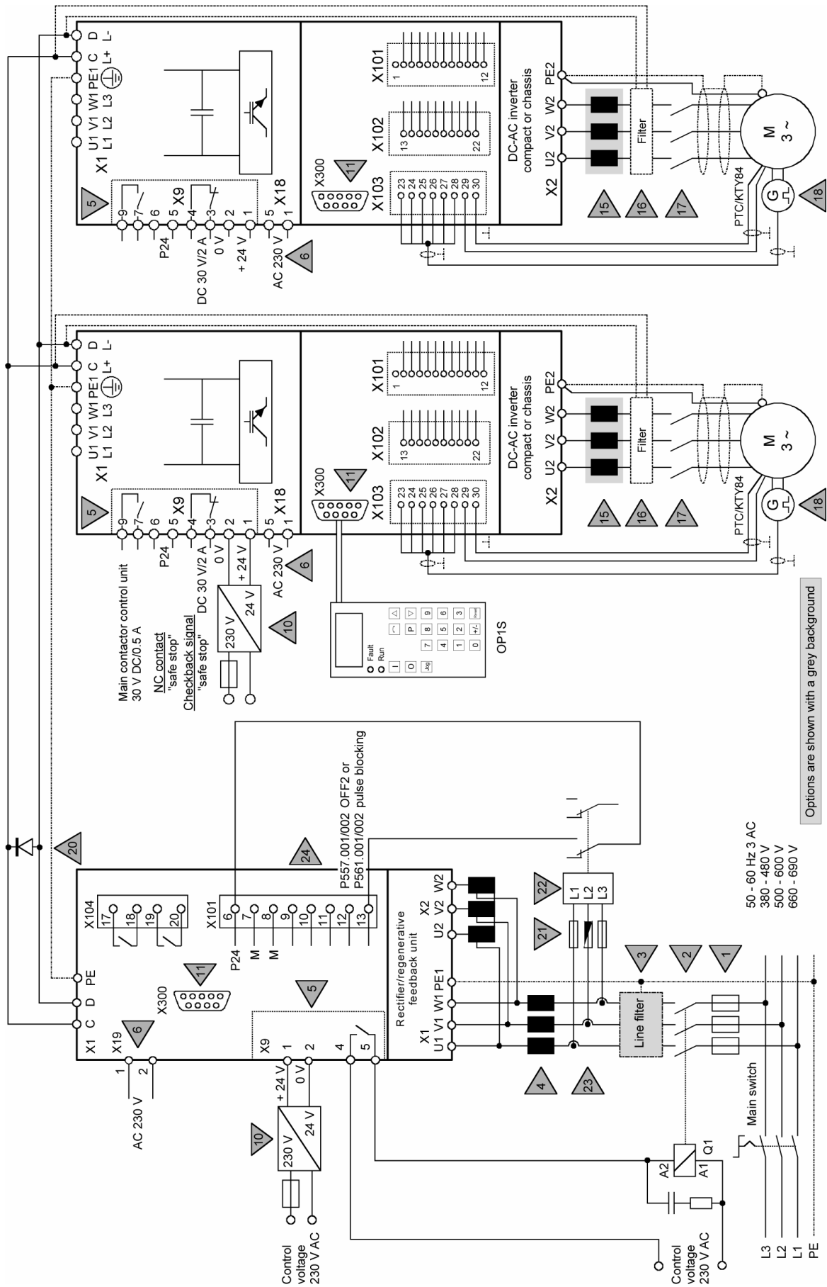
图 2-6 用整流/回馈单元的配置举例
