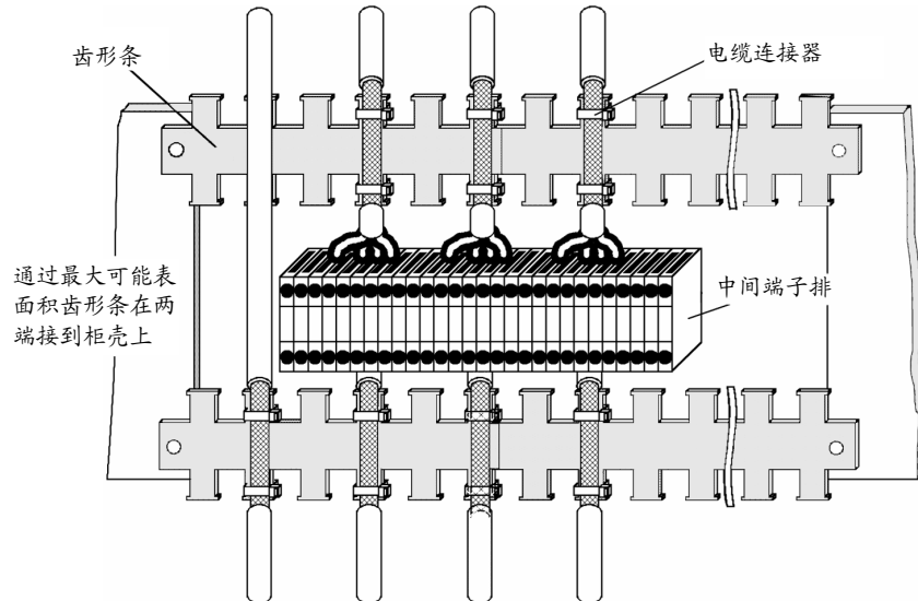
图 3-13 在柜中连接信号电缆屏蔽层
