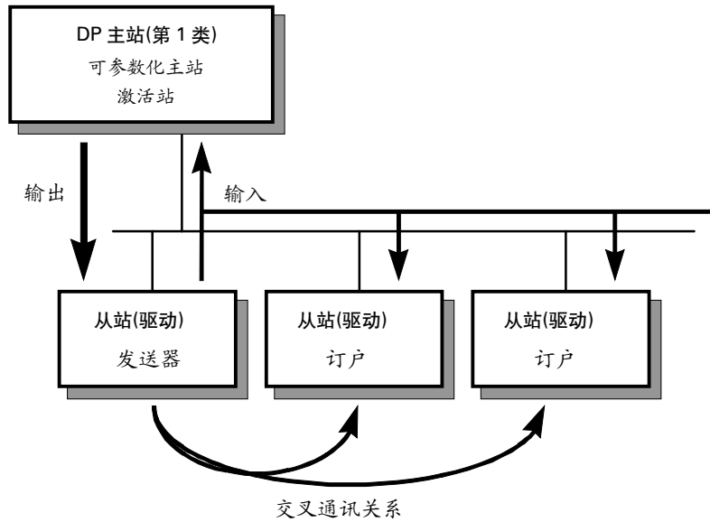
图 8.2-24 交叉通讯
