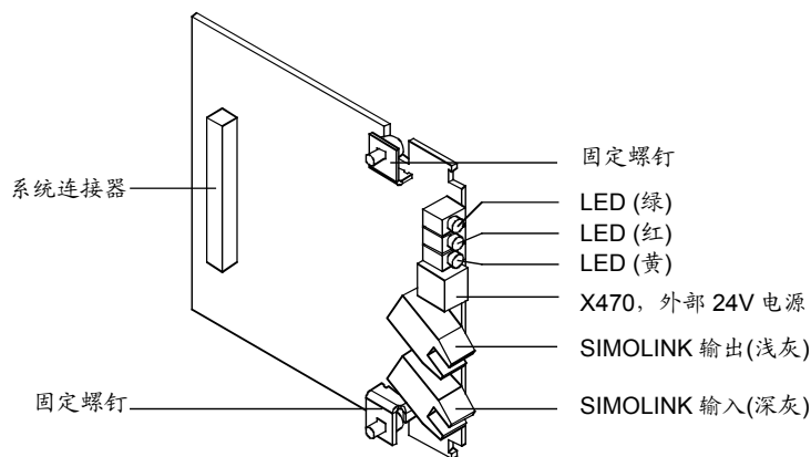
图 8.3-6 SLB 选件板(SIMOLINK 板)
