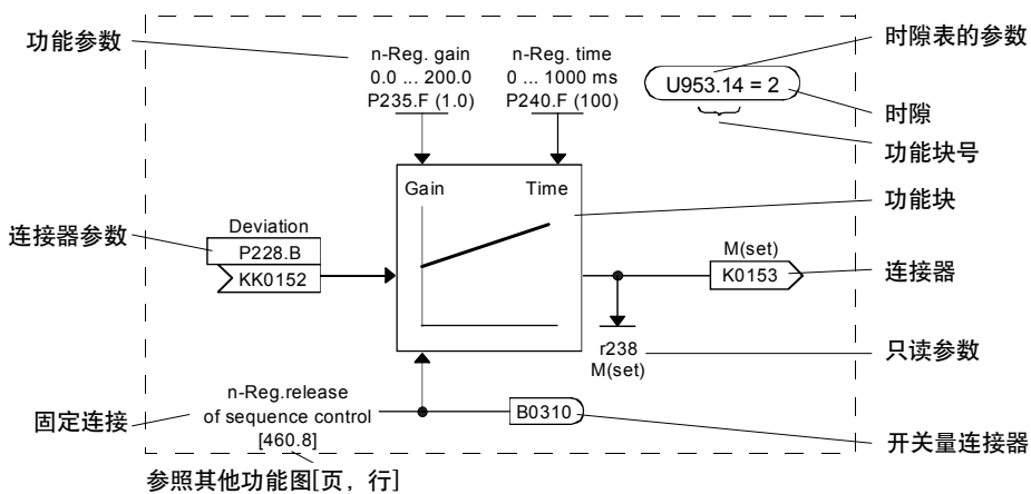
图 4-1 一个功能块
