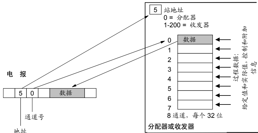
图 8.3-4 写数据
